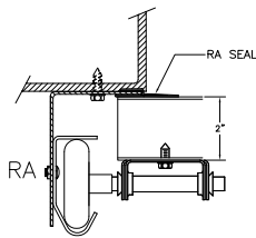
3" STEEL JAMB
